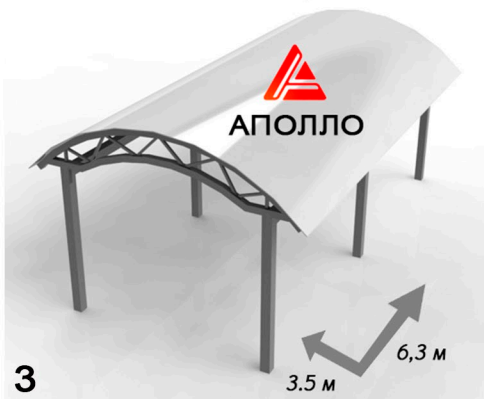
Навес арочный 3,5 х 6,3 м.
