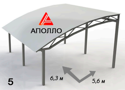
Навес арочный односкатный 5.6 х 6,3 м.
